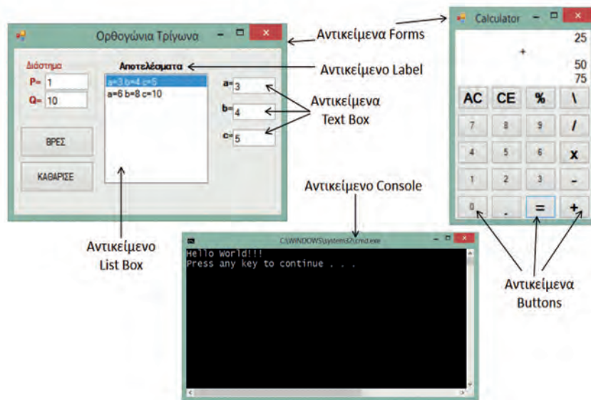
Εικόνα 2-5. Προγραμματιστικά αντικείμενα
